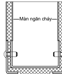
MẶT CẮT THANH ĐÁY MÀN
