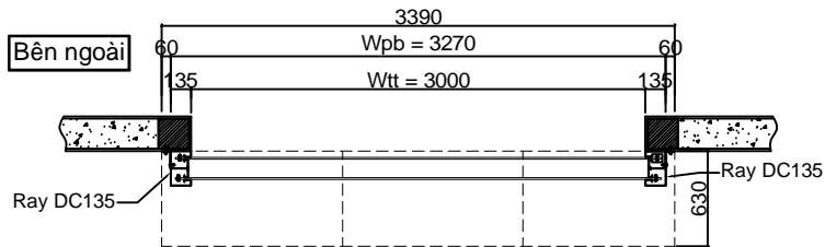
MẶT CẮT NGANG
