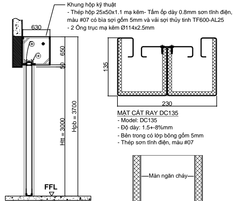
MẶT CẮT ĐỨNG
