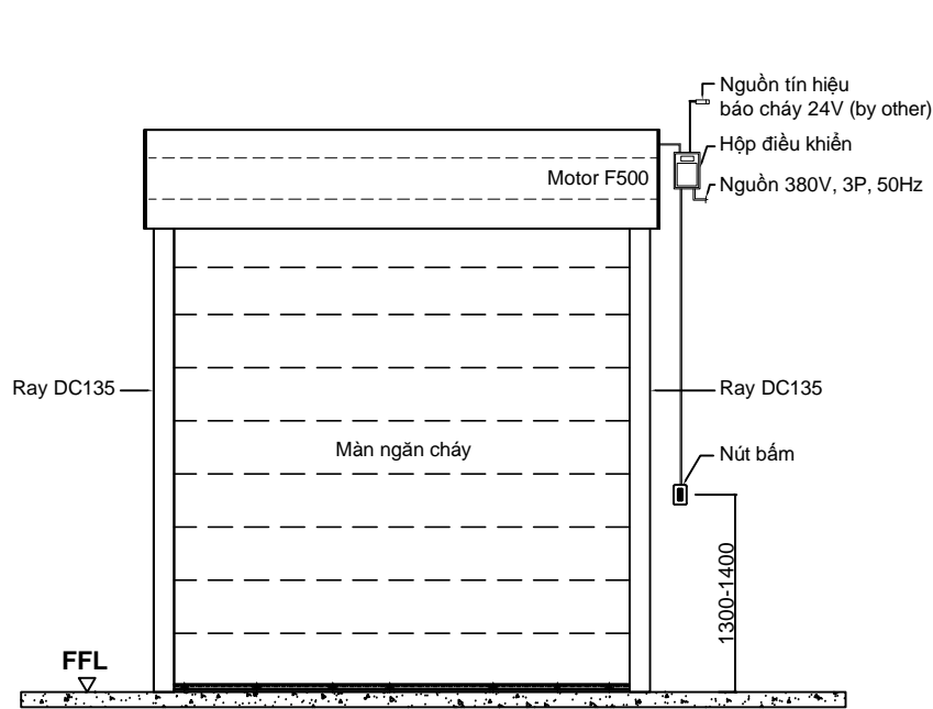
MẶT ĐỨNG
