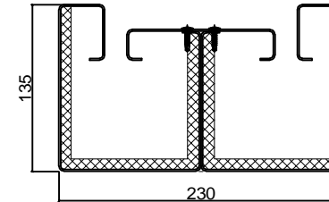
MẶT CẮT RAY DC135
