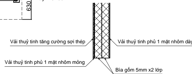
CHI TIẾT MÀN CỬA
