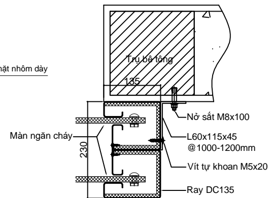
CHI TIẾT LẮP RAY DC135
